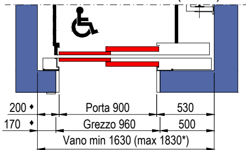
PIANTA VANO CORSA PORTE SENZA TELAIO (EI120)
