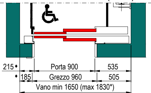
PIANTA VANO CORSA PORTE SENZA TELAIO (E120)
