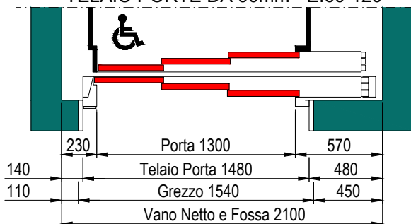
PIANTA VANO CORSA TELAIO PORTE DA 90mm - E160-120
