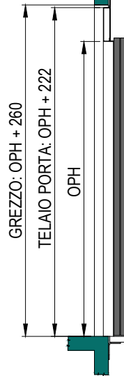
SEZIONE PORTA CON TELAIO DA 90mm (E160 - E120)
