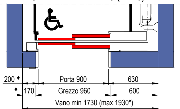
PIANTA VANO CORSA PORTE SENZA TELAIIO (EI120)
