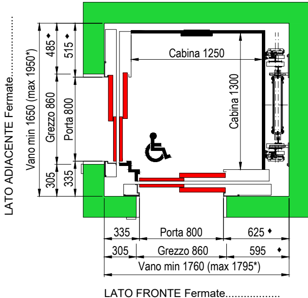
PIANTA VANO CORSA PORTE SENZA TELAIO (EI120)
