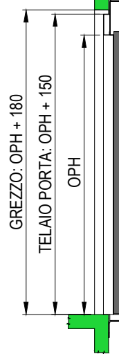
SEZIONE PORTA CON TELAIO DA 150mm
