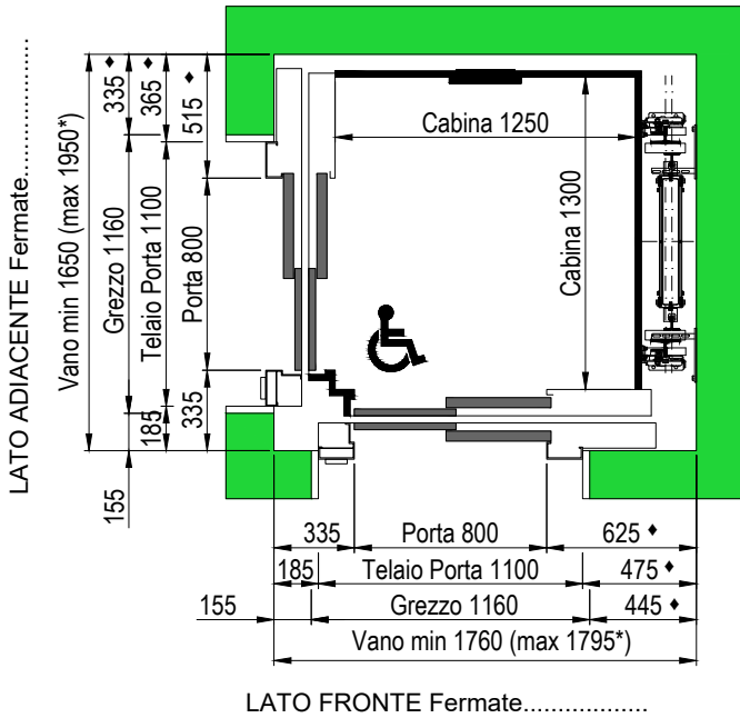
PIANTA VANO CORSA TELAIO PORTE DA 150mm
