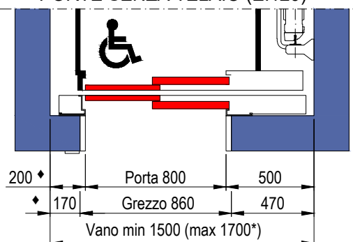
PIANTA VANO CORSA PORTE SENZA TELAIO (EI120)
