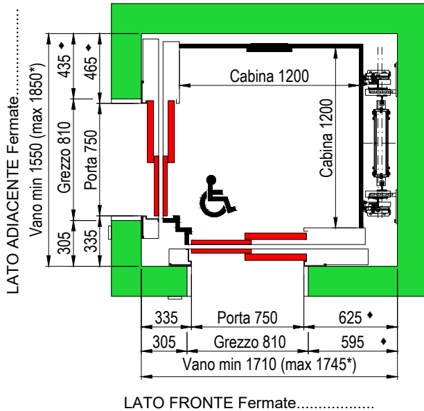
PIANTA VANO CORSA PORTE SENZA TELAIO (EI120)
