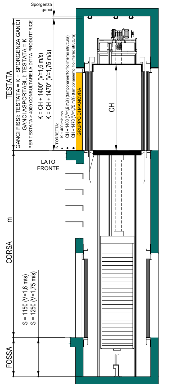
SEZIONE VANO CORSA
