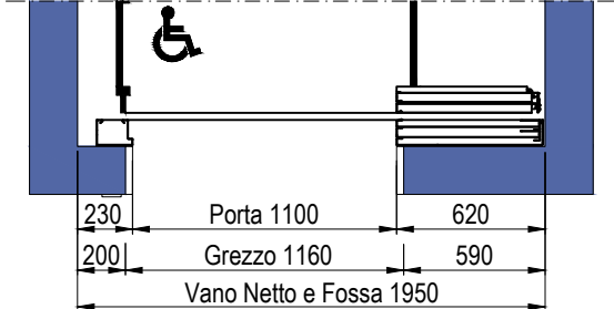
PIANTA VANO CORSA PORTE SENZA STIPITI - E1120
