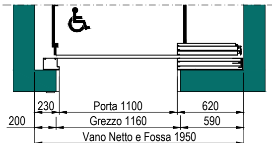
PIANTA VANO CORSA PORTE SENZA STIPITI - E1120
