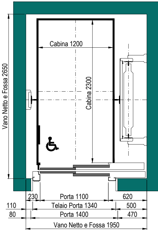
PIANTA VANO CORSA PORTE CO TELAIO DA 150mm
