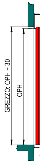
SEZIONE PORTA SENZA TELAIO (E1120)
