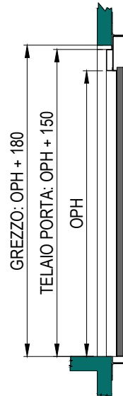
SEZIONE PORTA CON TELAIO DA 150mm
