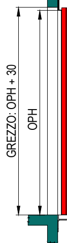
SEZIONE PORTE SENZA TELAIIO (EI120)
