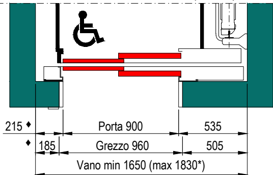
PIANTA VANO CORSA PORTE SENZA TELAIO (E120)
