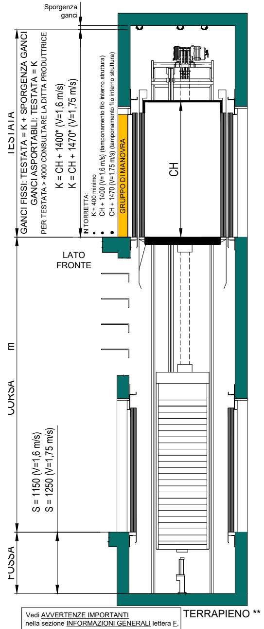
SEZIONE VANO CORSA
