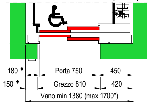
PIANTA VANO CORSA PORTE SENZA TELAIO (E1120)
