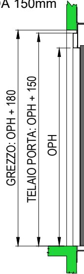
SEZIONE PORTE SENZA TELAIO (E1120)
