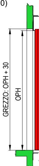
SEZIONE PORTE SENZA TELAIO (E120)
