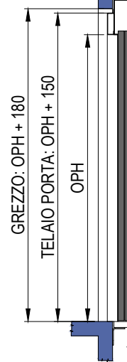
SEZIONE PORTE SENZA TELAIO (EI120)
